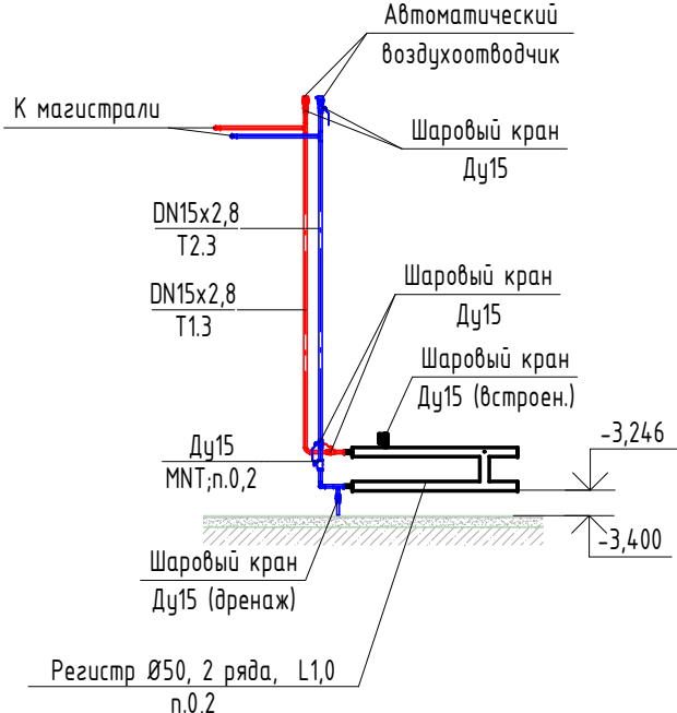
Узел подключения регистра в тамбуре на отм. ниже 0,000
