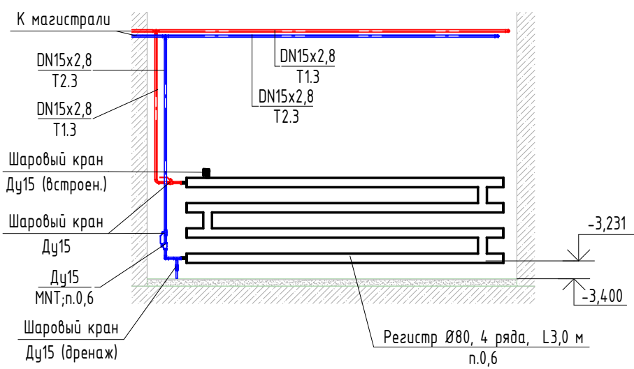
Узел подключения регистра в тех.помещении на отм. ниже 0,000
