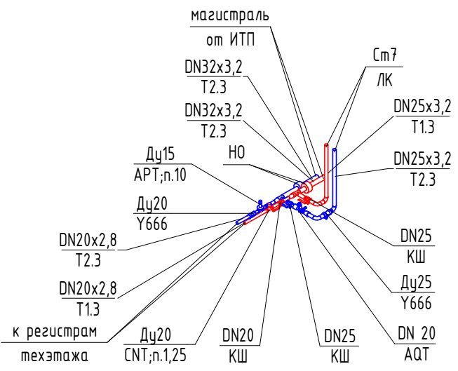
Узлы подключения стояка отопления ЛК и МОП техэтажа
